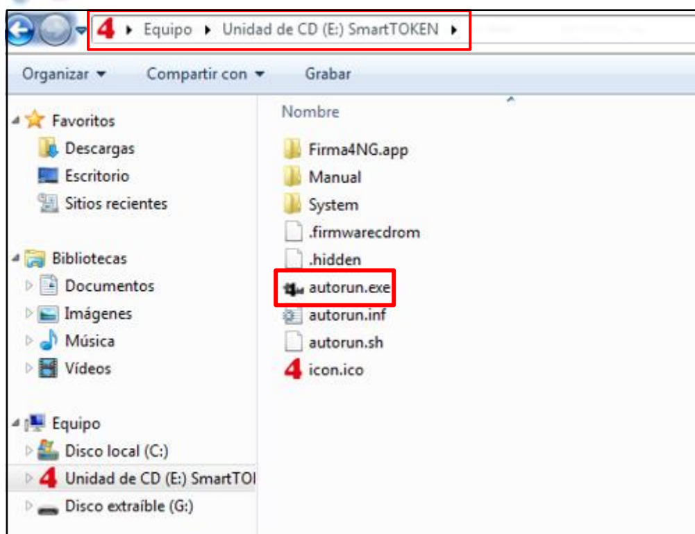
Figura 1: Autorun.exe
