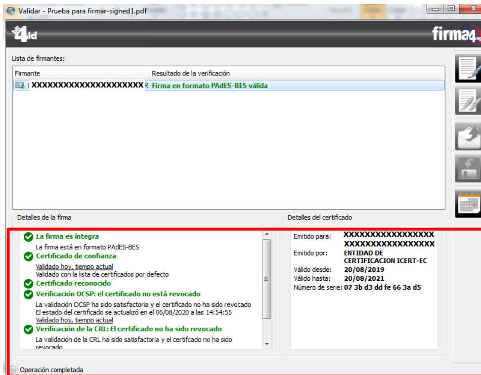
Figura 7: Operación satisfactoria.
