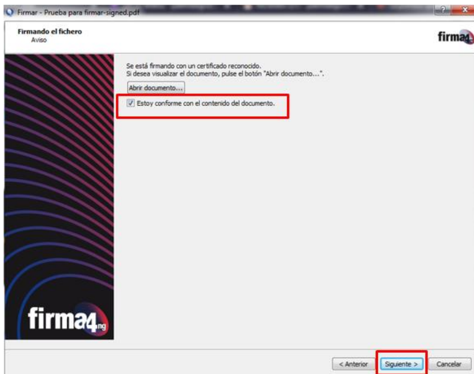
Figura 5: Check list
